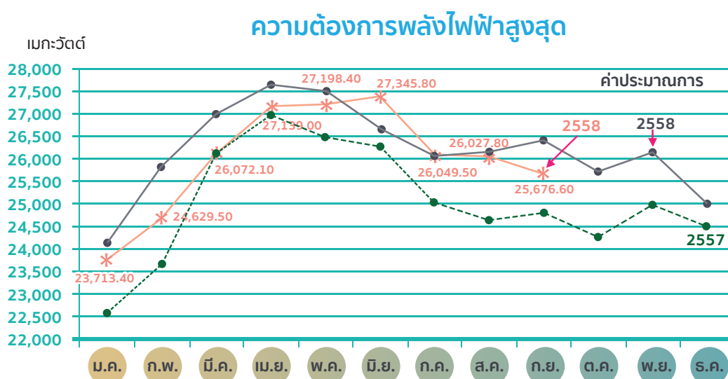
รูปที่ 1 แสดงความต้องการใช้พลังงานไฟฟ้าสูงสุดในปี 2558 (มกราคม - กันยายน 2558) ที่มา : กฟผ.
